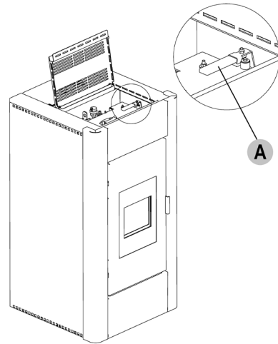
Fig. 19 - Hebel für die Reinigung der Rohrleitungen (Idro Prince 30-30 H2O)
