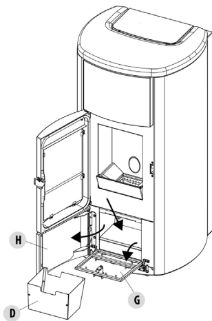
Fig. 14 - Entnahme Aschenlade
