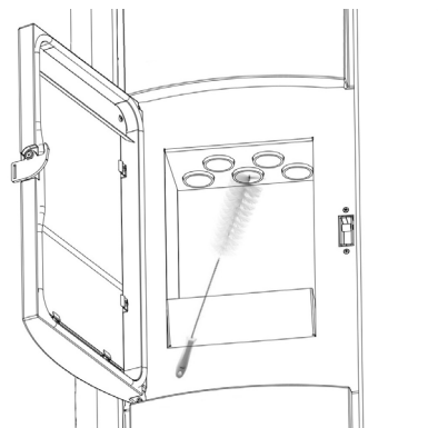
Fig. 20 - Reinigung der Rohrbündel
